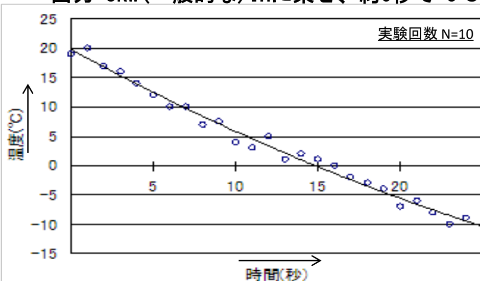
【 性能評価 (IH出力 1kW使用時) 】
