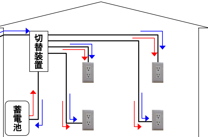
【 従来技術 】
